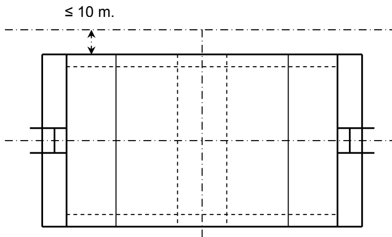
Figure 4 Distance minimale d'implantation des luminaires.
